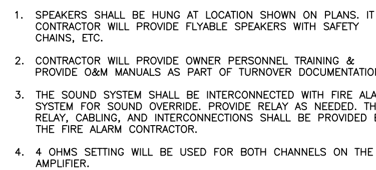
001.1 SOUND SYSTEM RISER SCALE: NONE
