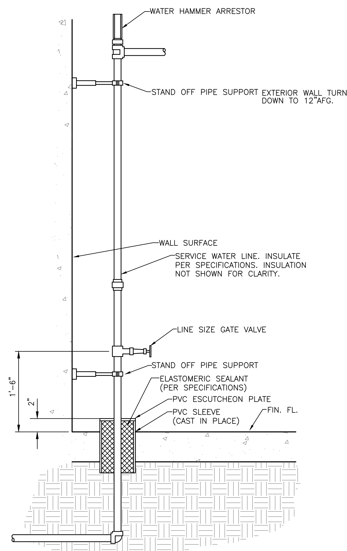
COLD WATER RISER DETAIL SCALE: N.T.S.
