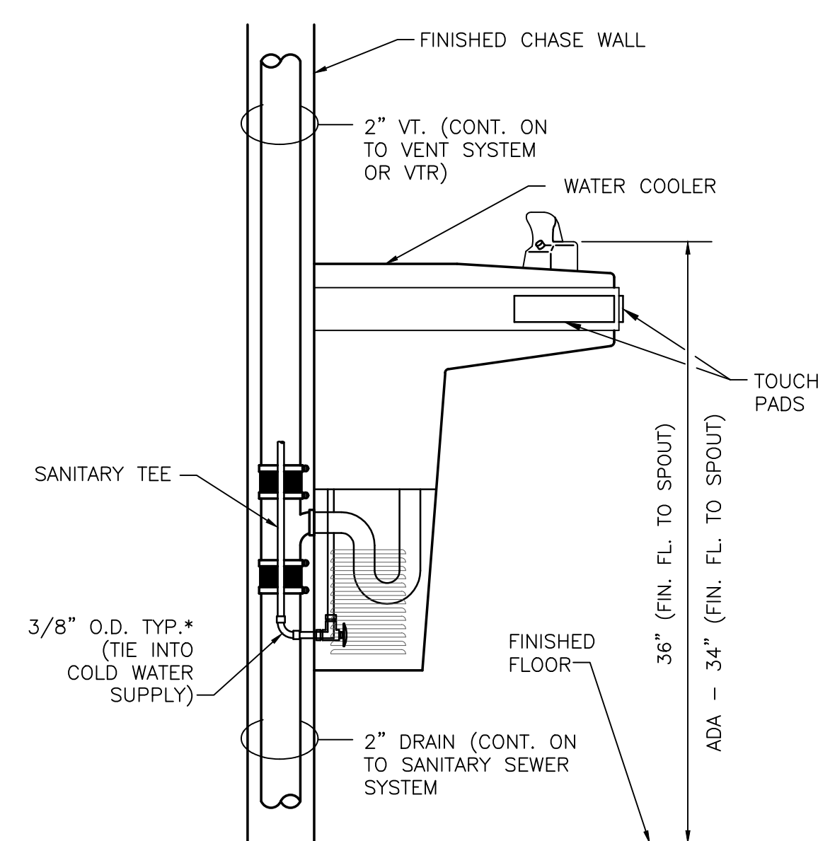
ELECTRIC WATER COOLER SCALE: N.T.S.
